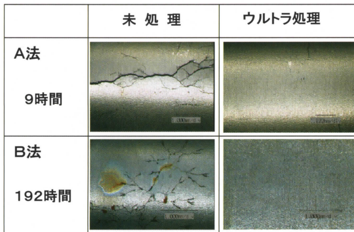
図2 応力腐食割れ試験(JIS G0576)
