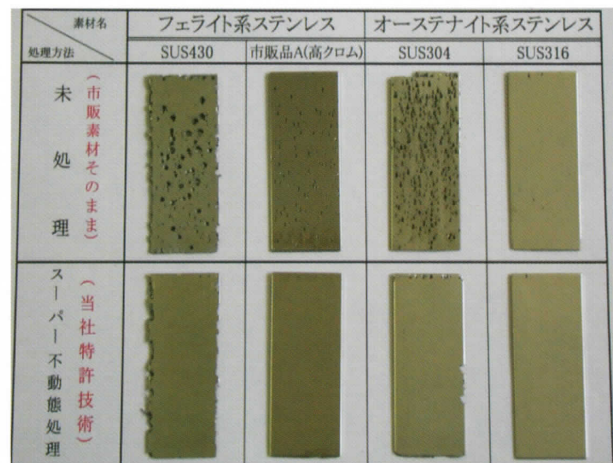
図3 孔食試験(JIS G0578)
