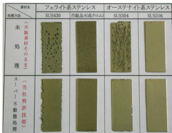
図3 孔食試験(JIS G0578)
