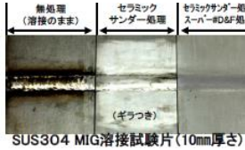
SUS304 MIG溶接試験片(10mm厚さ)
